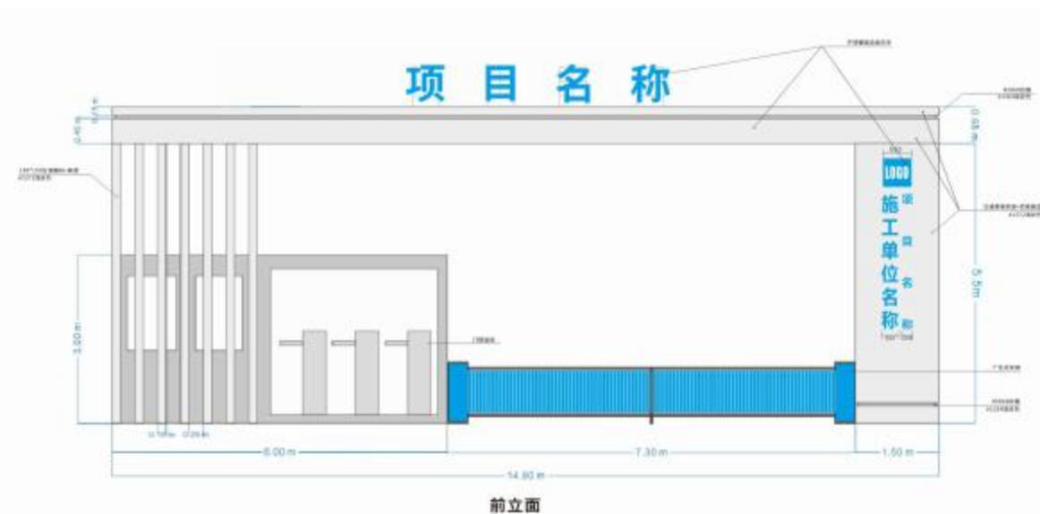
主大门立面图样式图 (具体项目、单位信息结合项目实际情况制定)
