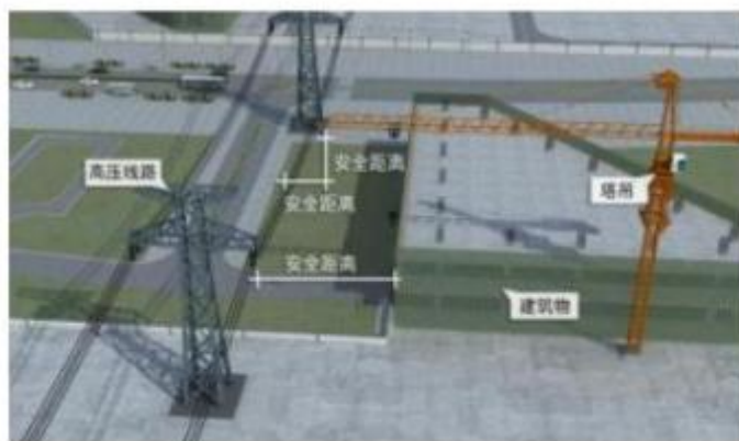
在建工程与外电路
