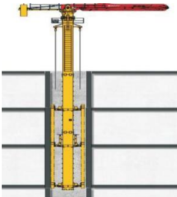
自升式布料机
