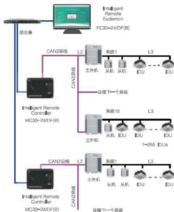
图 5-10 系统拓扑图片
