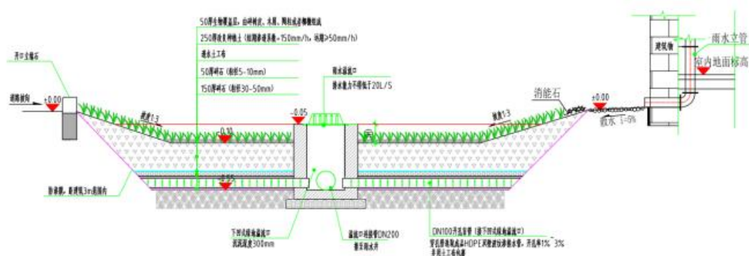
图5-2-7 下凹式绿地做法大样图
