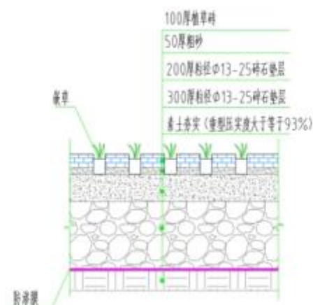
图5-2-8 透水植草砖做法大样图
