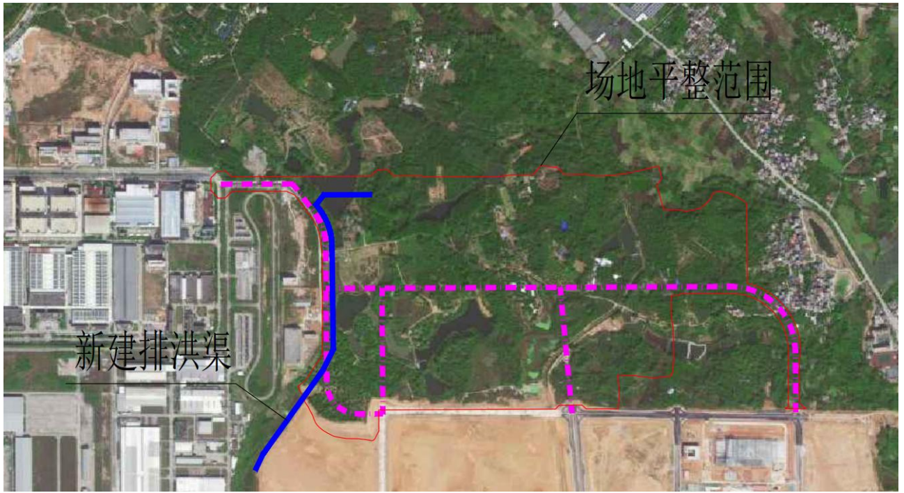
场地平整范围及新建规划排洪渠位置图
