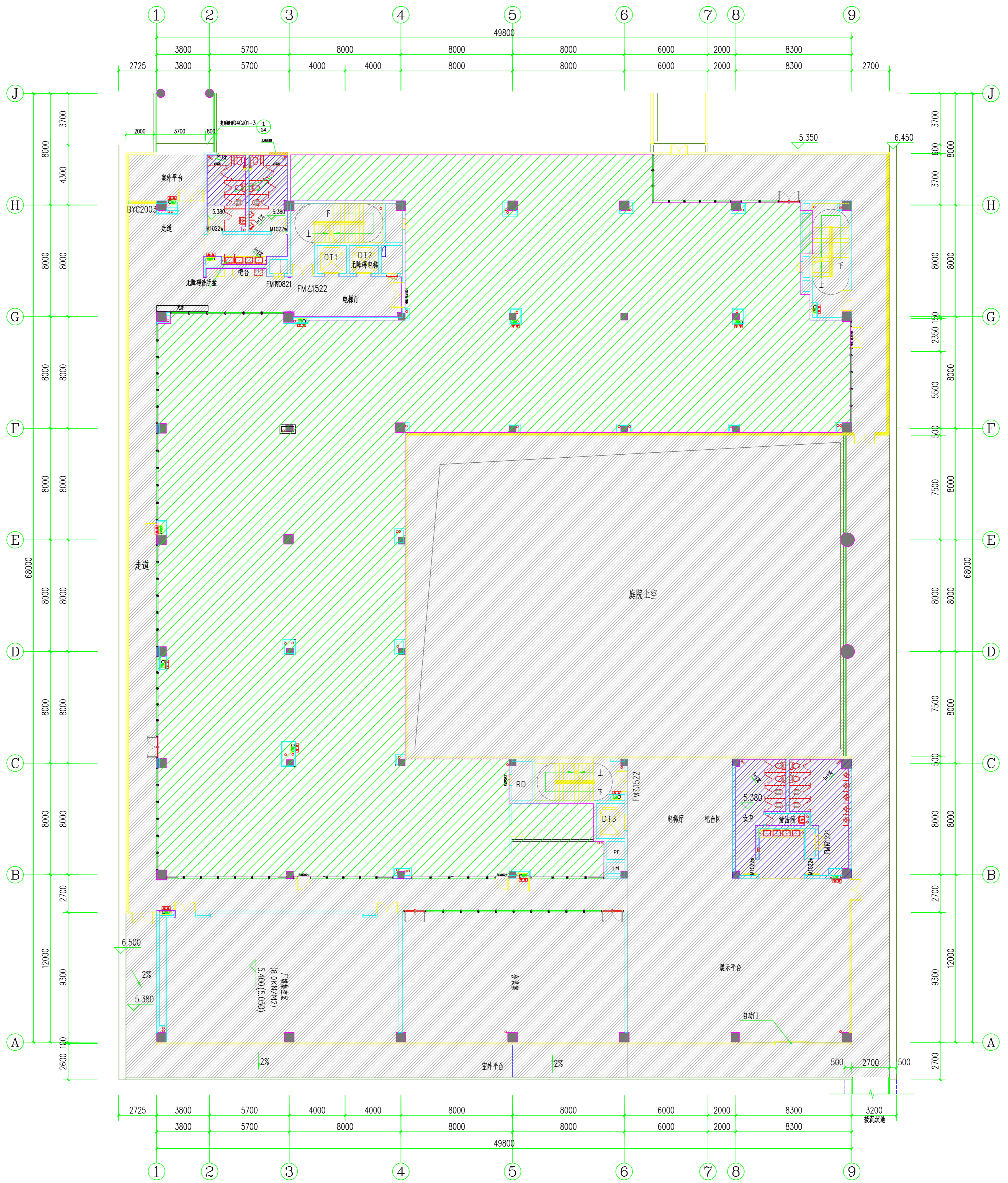
实验室布置需求提资平面图 1:150
